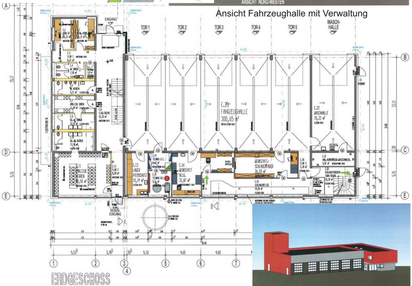
Grundriss Erdgeschoss
